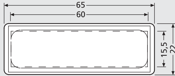
97-9-82033 Namensschild ohne Feder für Klappe nach außen aufgehend. Namensschildeinlage max. 60 x 15 x 0,5 mm, Ausstanzung 61 x 18 mm € 3,00
