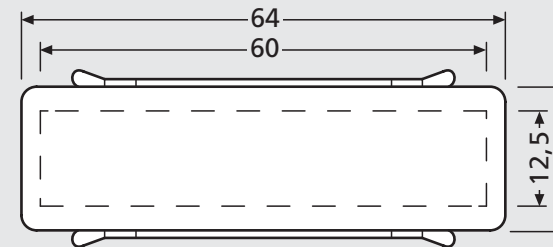
97-9-00303 Namensschild mit Feder Namensschildeinlage max. 60 x 12,5 x 0,5 mm, Ausstanzung 60 x 15 mm € 3,00
