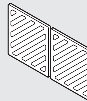
97-9-00094 Sprechgitter 75 x 80 mm für Modellgruppe 11/12, mit Nippel für Adapterbefestigung, ohne Schloss (2 St. erforderlich, siehe Abbildung), Ausstanzung 71,3 x 75,3 mm, Farben: braun, weiß, grau (bei Bestellung bitte Farbe angeben) inkl. 4 Befestigungsclips Ø 12 mm € 7,10
