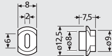
97-9-82035 Namensschildsperre passend zu 97-9-82033 € 1,10
