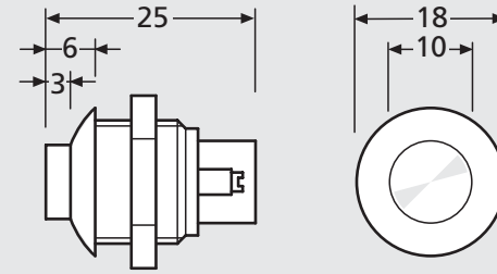
97-9-85062 Lichtknopf Lira, Rand schwarz, Drücker rot Ausstanzung 15,5 mm € 12,10
