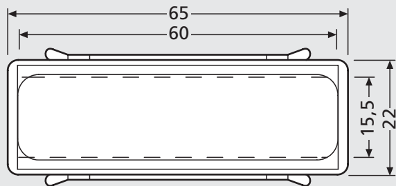
97-9-00302 Namensschild mit Feder für Einbau in Türen, Namensschildeinlage max. 60 x 15 x 0,5 mm, Ausstanzung 61 x 18 mm € 3,00
