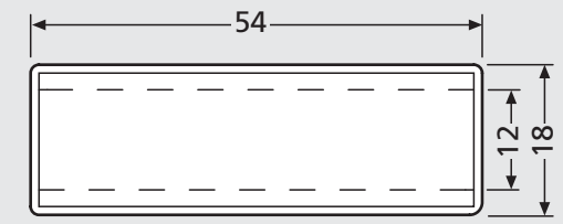
97-9-82014 Namensschild für Durchwurfhals Namensschildeinlage max. 50 x 12 x 0,5 mm, Ausstanzung 50 x 14 mm € 3,00
