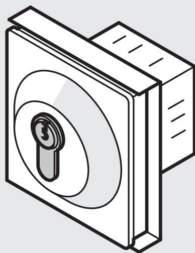
97-9-00206 Funktionsmodul in massiver ALU-Ausführung für Steuerung von Garagen- und Rolltoren usw. mit Taster 2-polig (max. 48 V) vorgerichtet für baus. Profilhalbzylinder L = 26, Schließnase 8-fach verstellbar, nach DIN mit ca. 40 mm Gesamtlänge. Ausstanzung 71,3 x 75,3 mm, Farben: braun, weiss, grau (bei Bestellung bitte Farbe angeben). € 149,60
