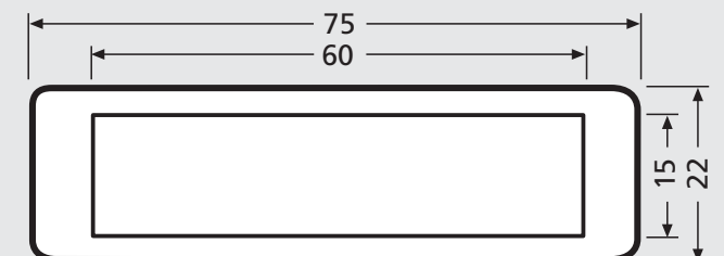
97-9-82016 Namensschild 92, 75 x 22 mm glasklar oder mit grauem Rand (bei Bestellung bitte Farbe angeben), Namensschildeinlage max. 60 x 15 x 0,5 mm, Ausstanzung 71 x 19 mm € 3,00
