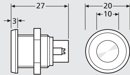
97-9-85027 Klingeltaster Lira, Rand und Drücker ALU silber Ausstanzung Ø 15,5 mm € 16,70
