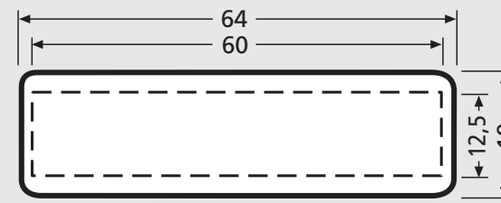
97-9-82019 Namensschild ohne Feder zum Einklipsen Namensschildeinlage max. 60 x 12,5 x 0,5 mm, Ausstanzung 60 x 15 mm € 3,00
