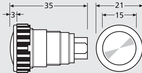
97-9-85148 Edelstahl-Klingelknopf, Antivandalismus RS4 , Ausstanzung Ø 18,5 mm € 26,30
