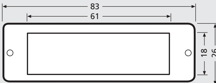
97-9-00212 ALU-Namensschildrahmen außen, Antivandalismus. Namensschildeinlage max. 74 x 23 x 0,5 mm EV 1 R 14 € 10,40 14,40
