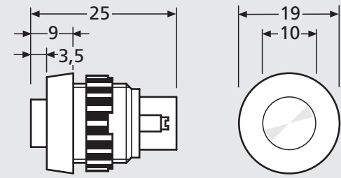
97-9-85024 Klingelknopf Rafi, Rand schwarz erhöht, Drücker weiß, Ausstanzung 15,5 mm € 5,50
