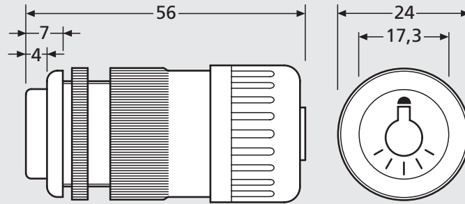
97-9-85063 Lichtknopf Grothe, Rand braun, für Kleinspannung, optional beleuchtbar mit Glühbirne 97-9-85036, mit hinterer Abdeckung, Ausstanzung Ø 21,0 mm € 24,00
